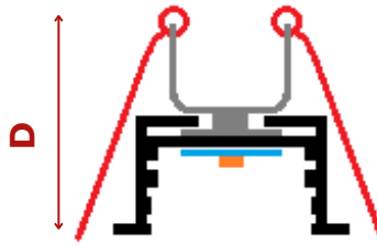
CONJUNTO MONTADO
