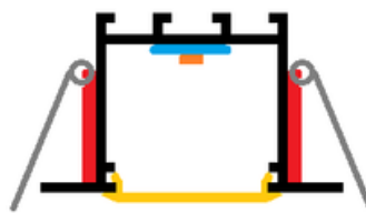
CONJUNTO MONTADO
